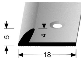
BP 70 bito Abschlussprofil 18 x 5 x 4 mm Art. 3038103 (Silber) | 3038104 (Sand)
