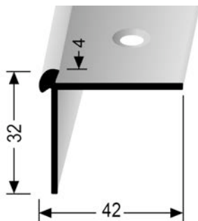
BP 69 bito Außenecke 42 x 32 x 4 mm, doppelt versenkt gebohrt Art. 3036220 (Silber) | 3036221 (Sand)
