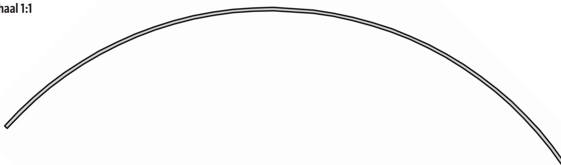
Buigsjabloon aluminium stroken houder ster Schaal 1:1
