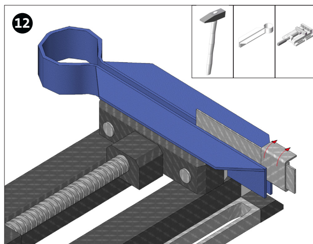
Uitstekende kanten ombuigen. (stap 3)
