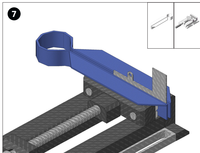
Werkstuk zoals afgebeeld in de buighulp spannen. In 4 stappen ombuigen.
