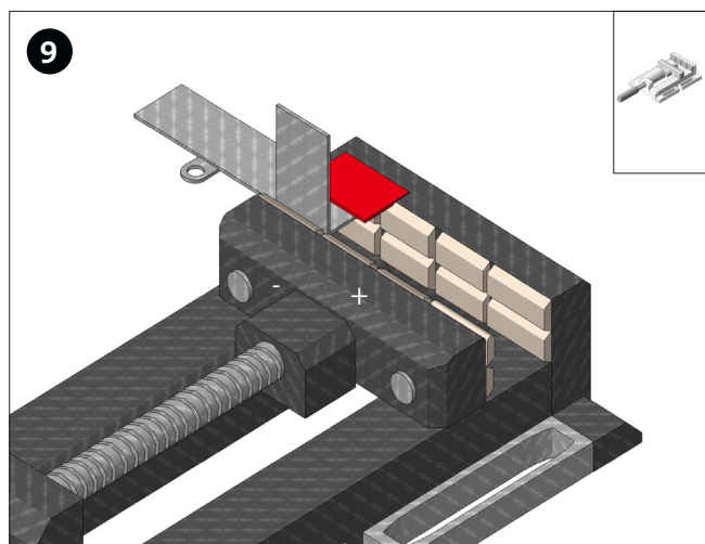
Buighulp (20 x 15 x 1 mm) zoals afgebeeld in het werkstuk plaatsen (stap 2). Tip: buighulp mag niet breder zijn dan het fluit stukje.
