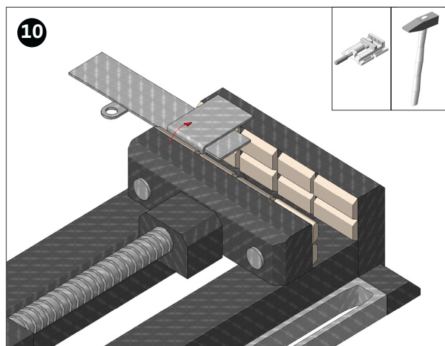
Mondstuk zoals afgebeeld ombuigen. (stap 2)
