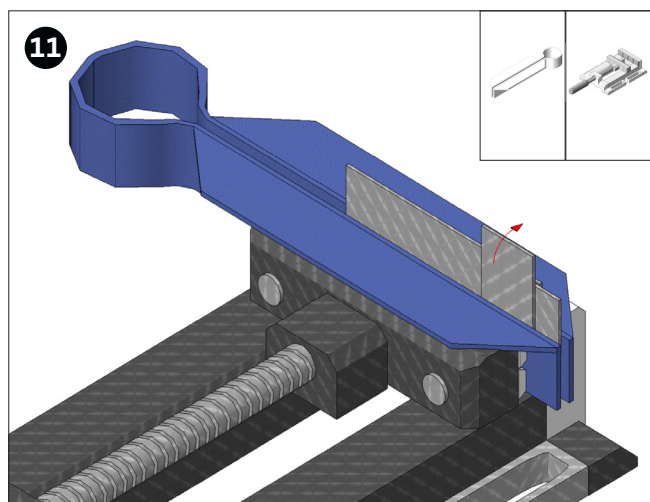
Werkstuk zoals afgebeeld in de buighulp spannen. (stap 3)
