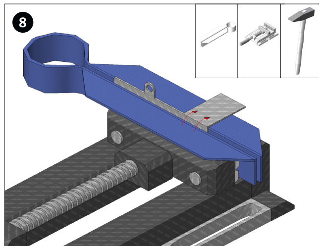
Mondstuk zoals afgebeeld ombuigen. (stap 1)
