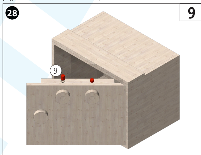
Introducir los imanes de barra (9) en el orificio. OJO: ¡Hay que asegurarse de que los polos de los dos imanes apunten a la misma dirección!
