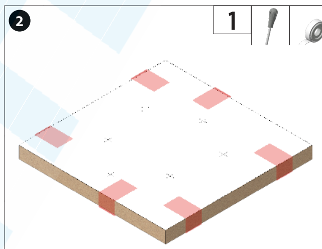
Sjabloon (A) op de grondplaat (1) plakken en de schroefposities voorstellen.
