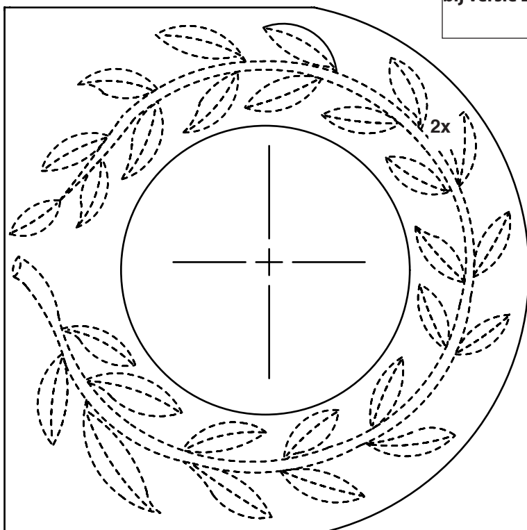
Sjabloon plankje voor bloemen schaal 1:1 versie 3
